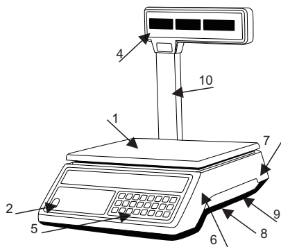
Рис. 1. Весы торговые электронные «М-ER 327-15.2», «М-ER 327-30.5», «М-ER 327P-15.2», «М-ER 327P-30.5»
