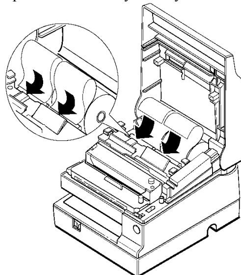
Рисунок 9 Подача бумаги в принтер
