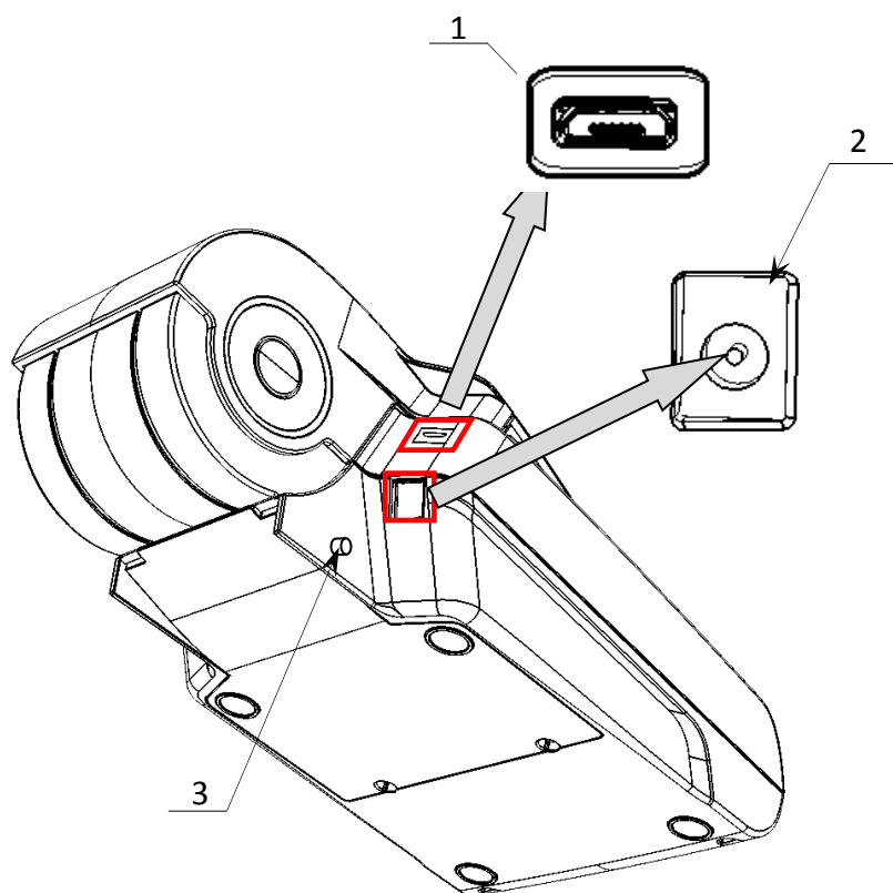
Рисунок 2. Вид сзади/снизу/слева
