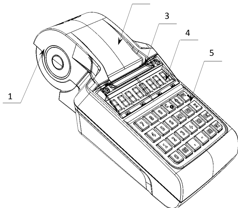
Рисунок 1. Вид спереди/сверху/слева
