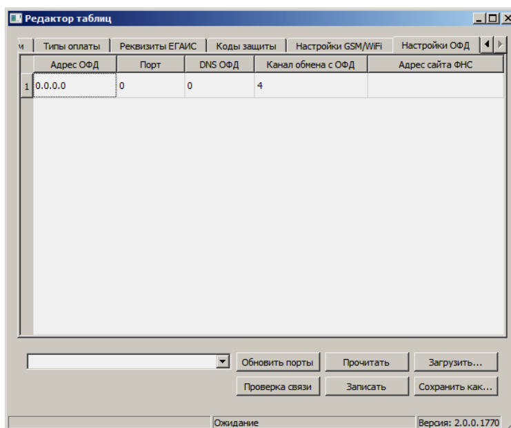
Рисунок 15. Вкладка «Настройки ОФД»
