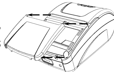
Рисунок 3. Крышка отсека для ФН отделена от корпуса ККТ
