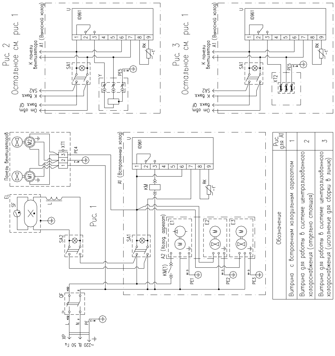
Схема электрооборудования витрины средне- и высокотемпературной "Связь 180" ВС (ВВ) (модели с встроенным и выносным холодом на фреоне R22)
