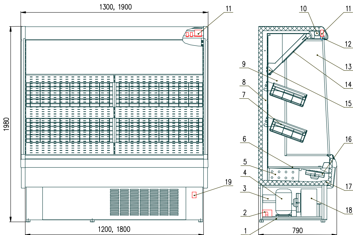
Рис. 16. Схема витрины «СВИТЯЗЬ П» ВВ:
