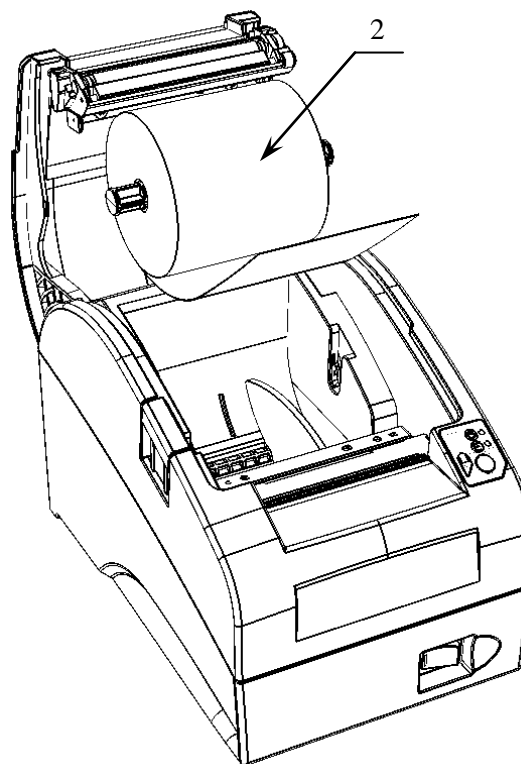
Рисунок 11. Установка ЧЛ.
